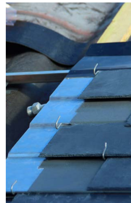
1. Systeem met haak
